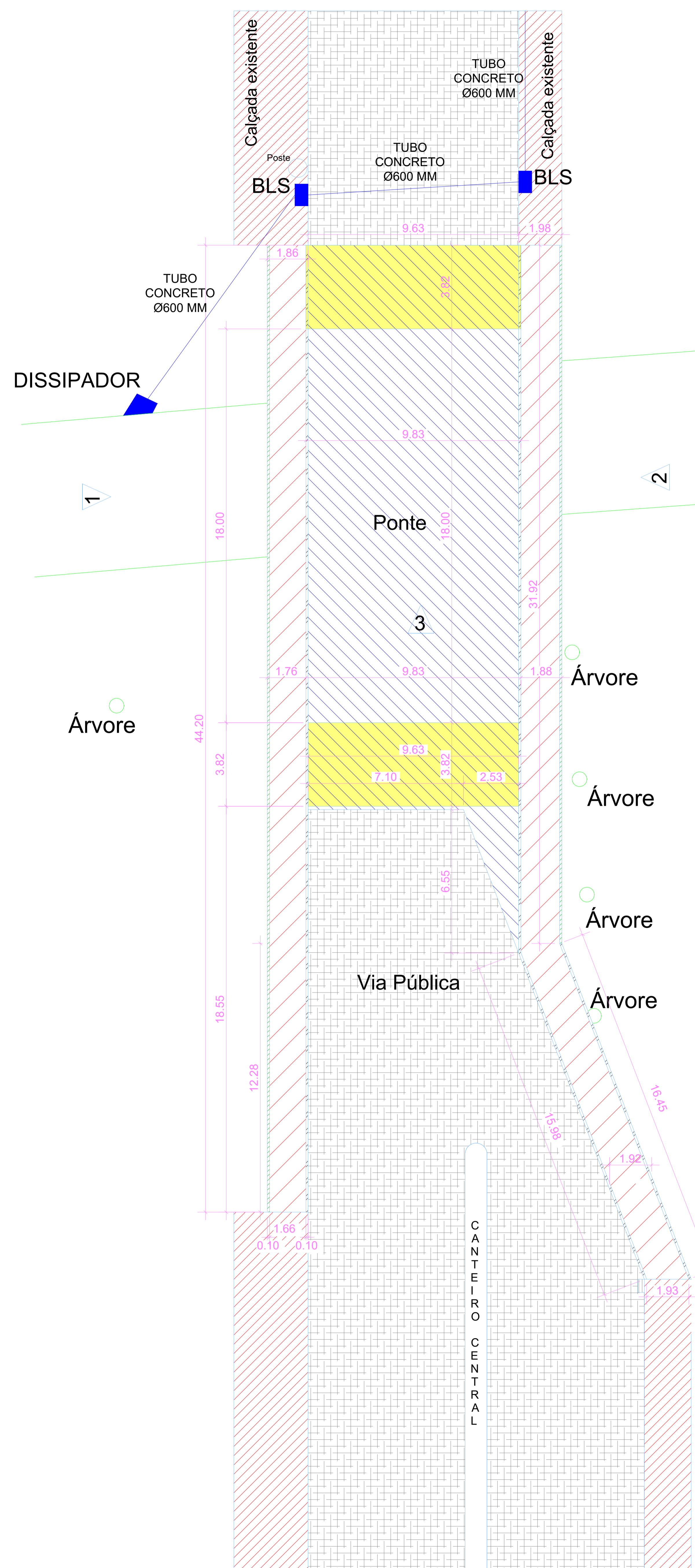
2 Situação Pretendida 1 : 100
