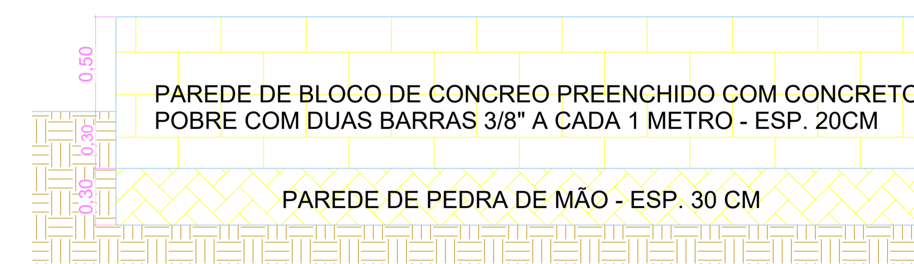
6 Muro 1:20
