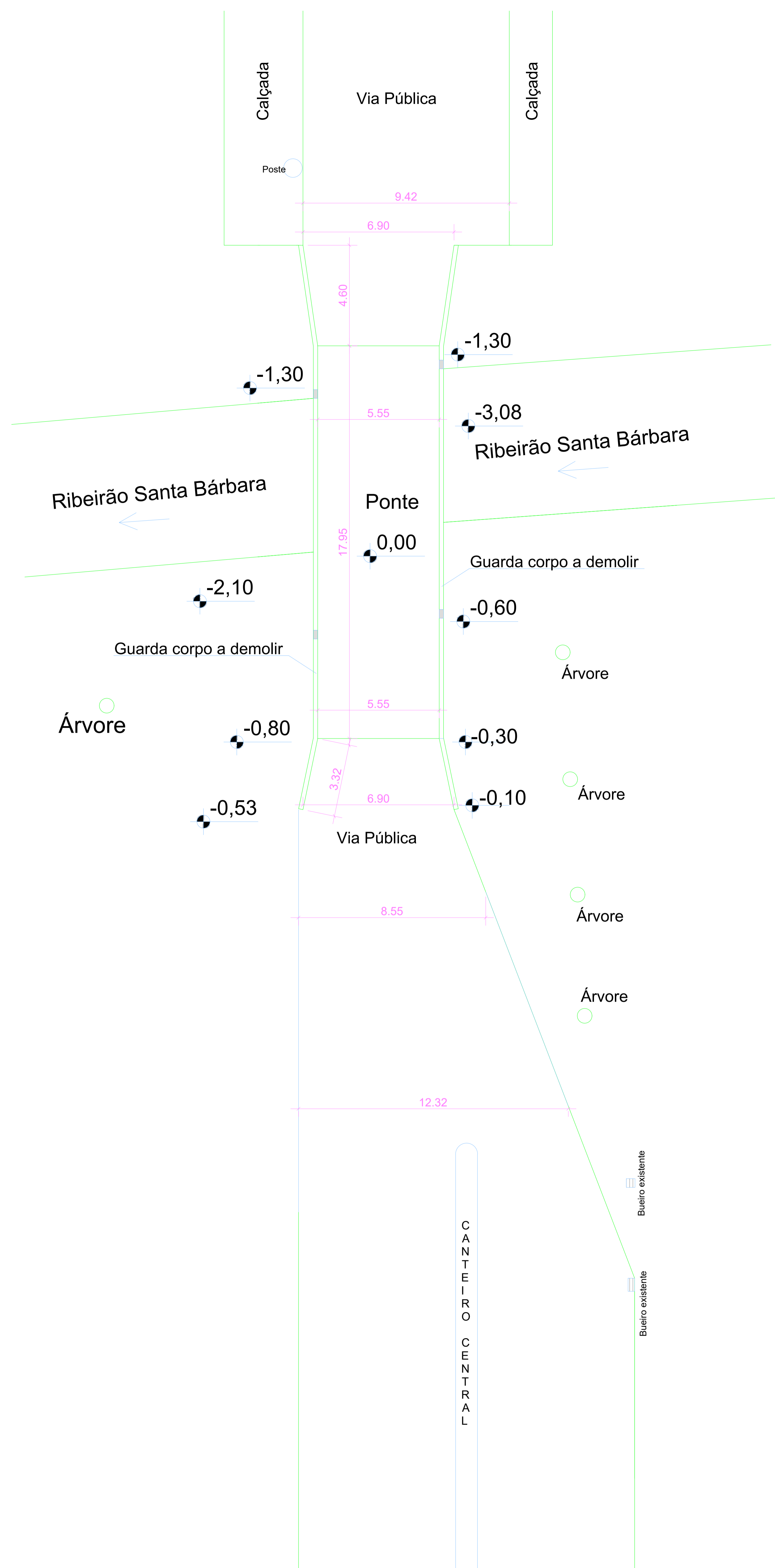
1 Situação Atual 1 : 100
