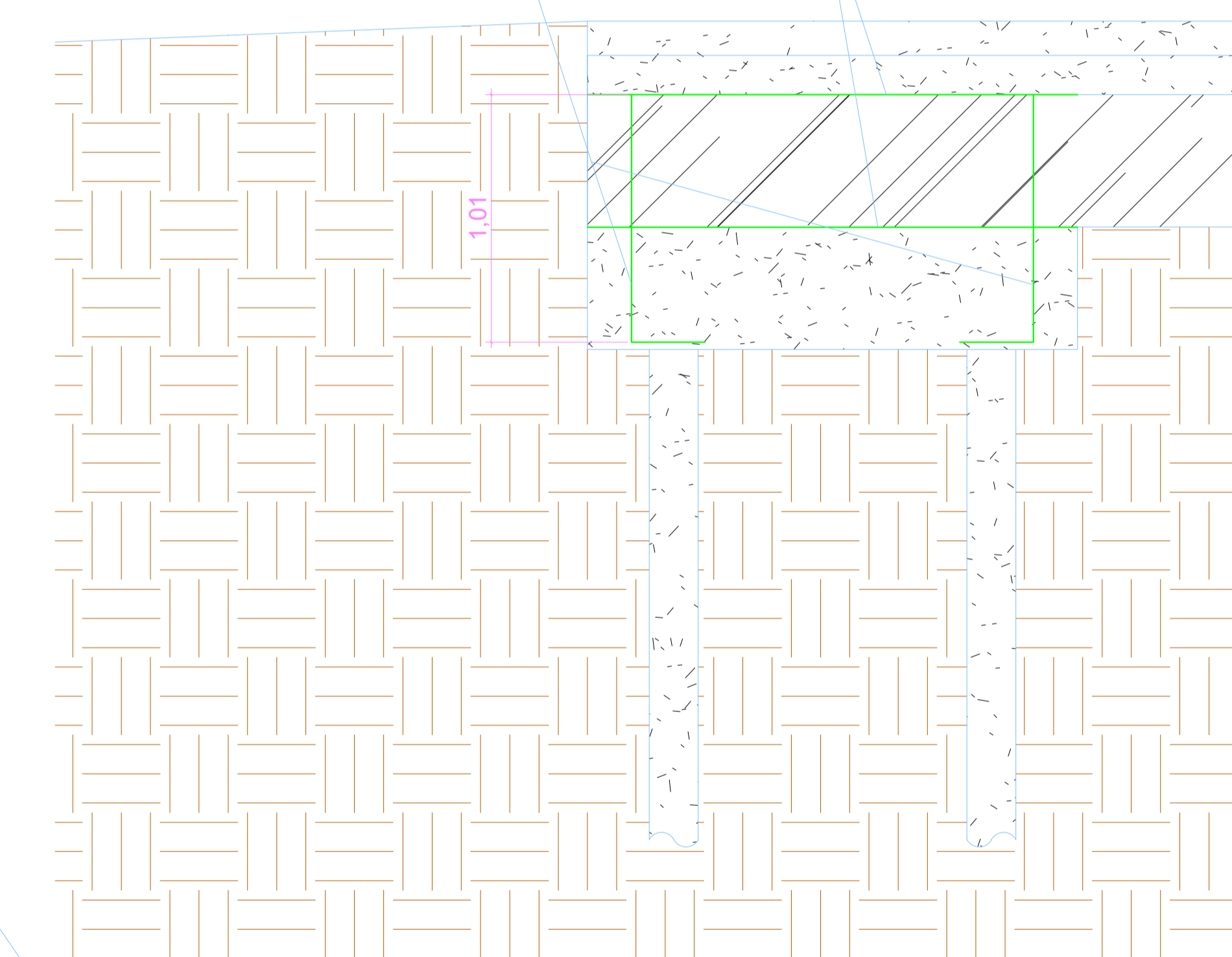
9 Detalhe 1 1:20
