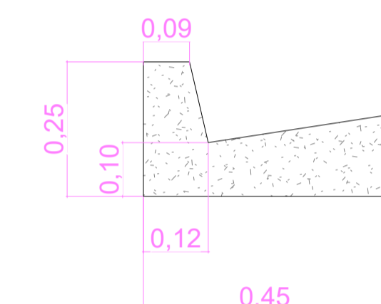
5 Sarjeta e Meio-fio 1:10
