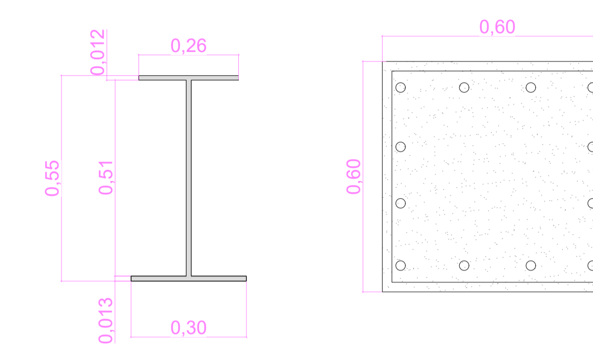
4 Vigas 1:10
